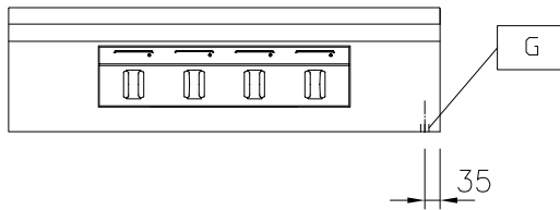
Zij aanzicht
